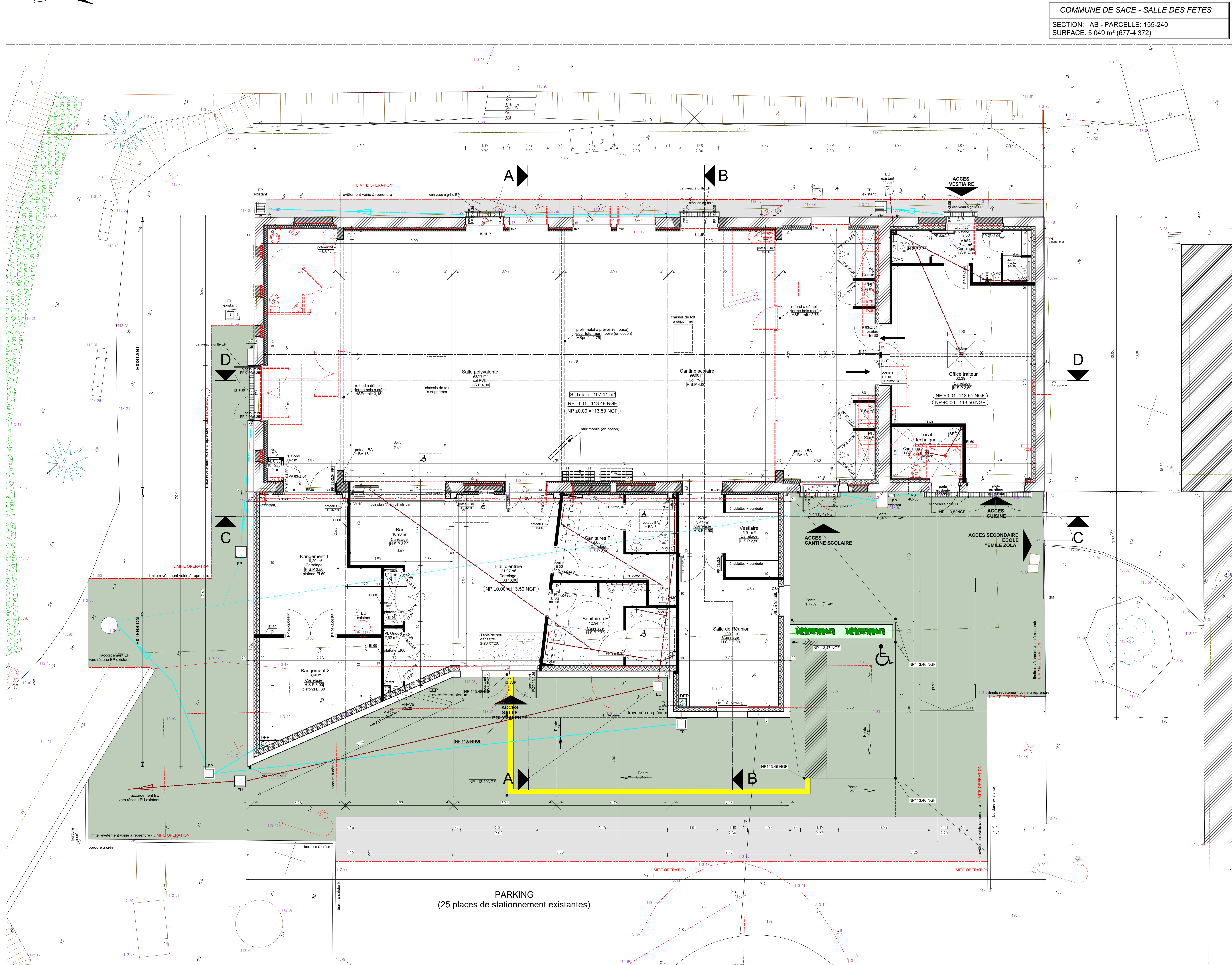
PLAN DE MASSE/RdC Echelle 1/500ème
